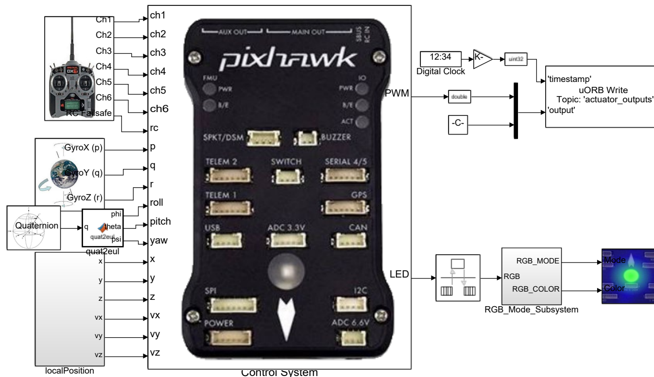
图. e8_1_HIL.slx截图
