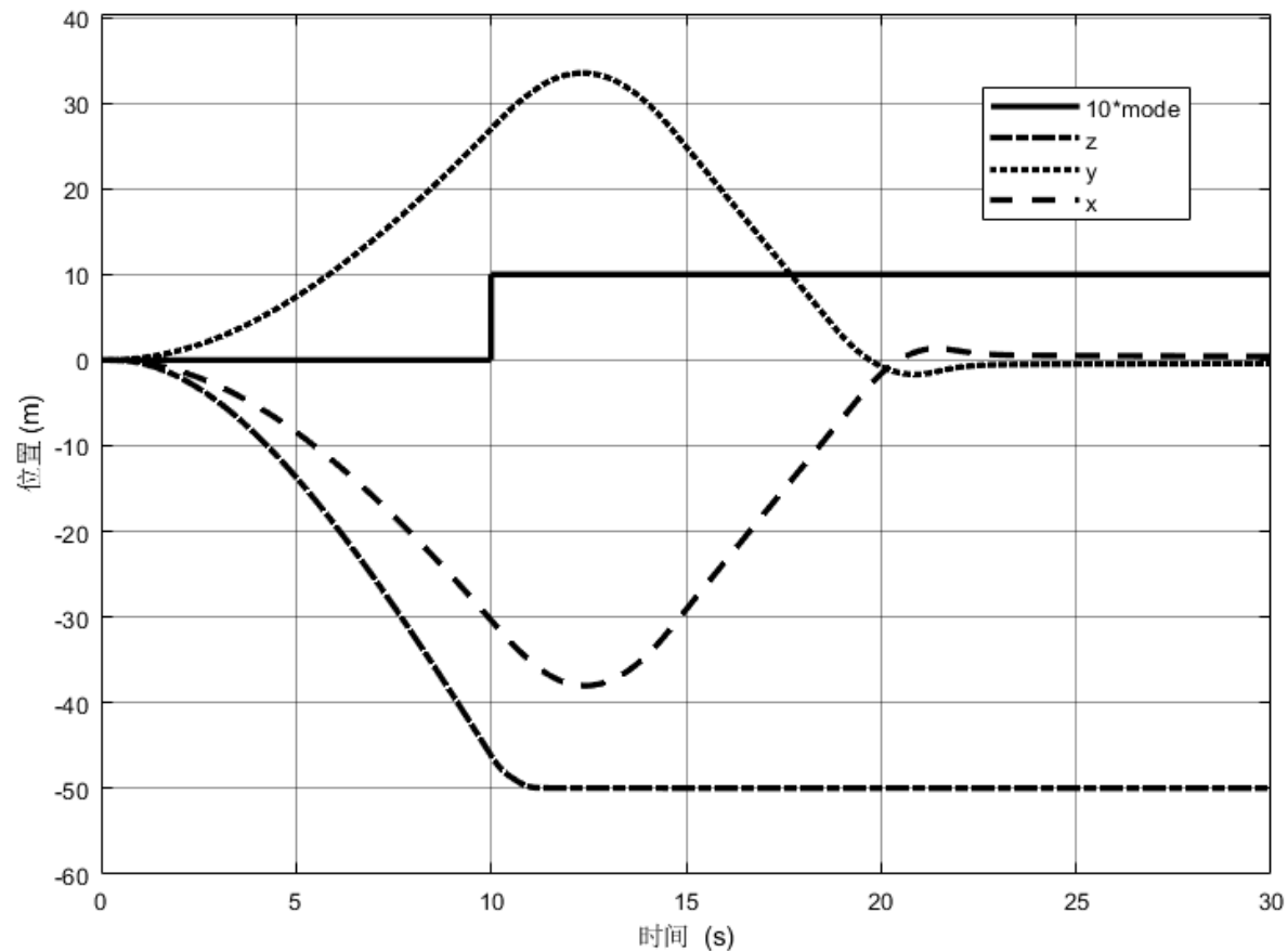
图. 手动模式下返航
