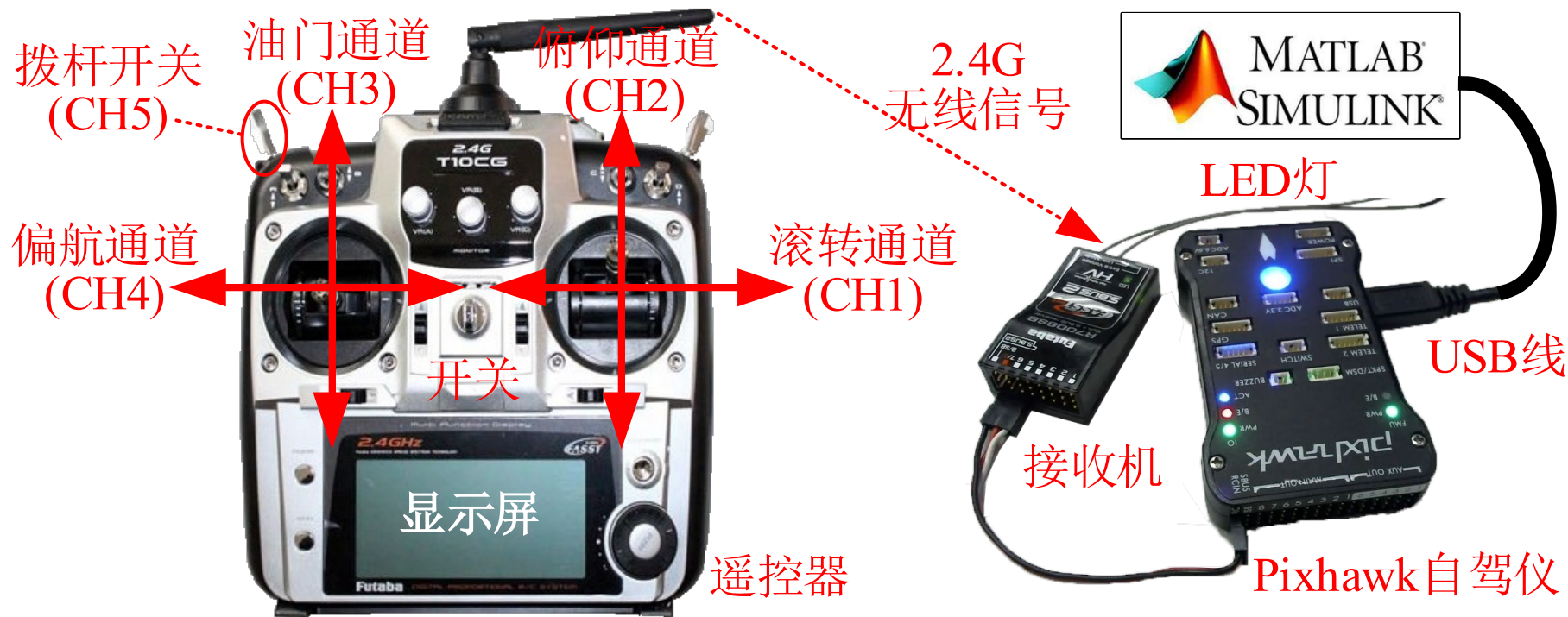
硬件连接图
